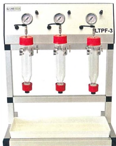
Ukázka tlakové filtrace LTPF-3
