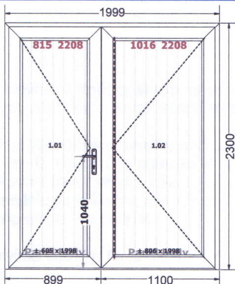
Pohled zevnitř, dveře otvíravé ven, levé hlavní křídlo
