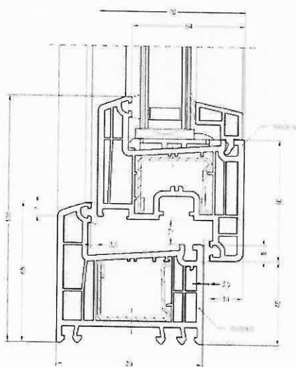
Detaily profilů
