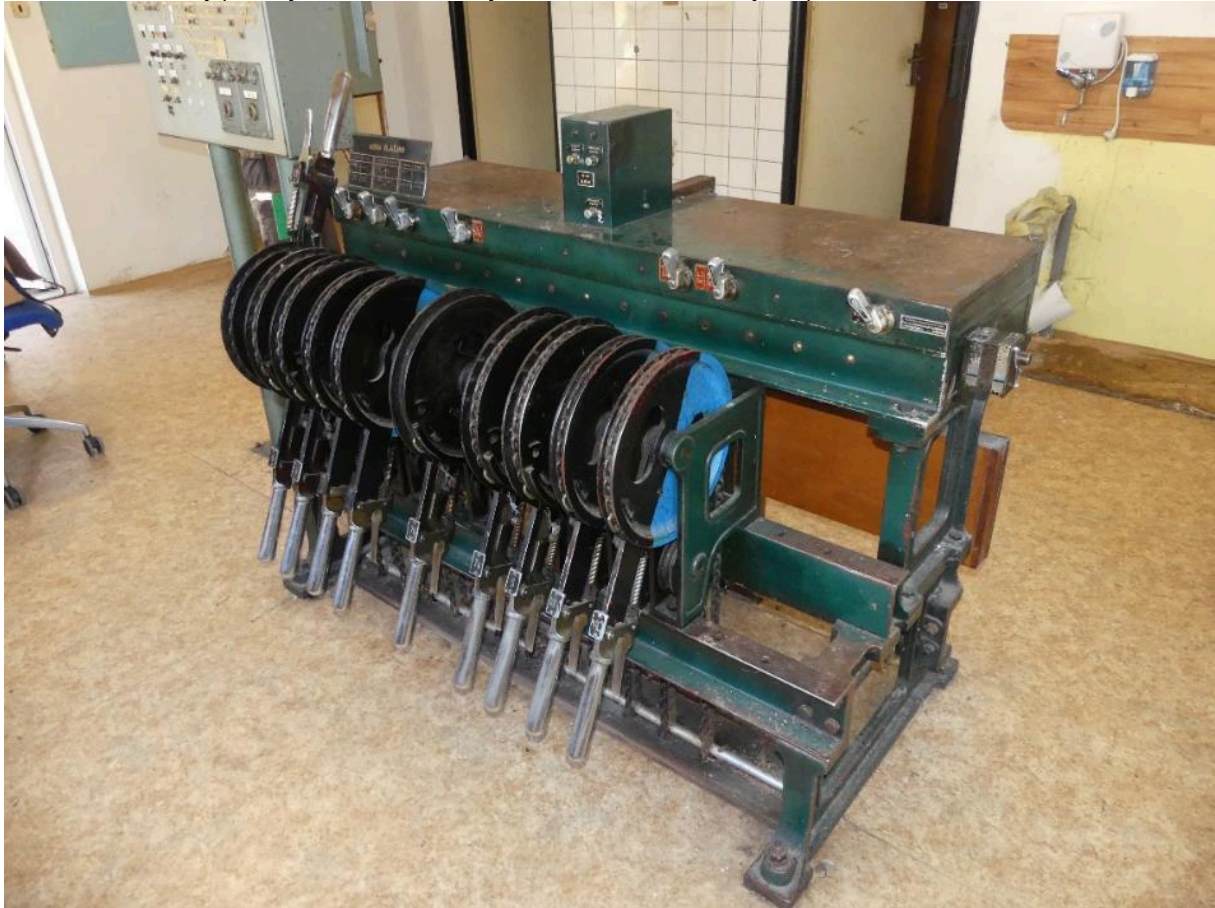
Ústřední stavědlový přístroj vzoru 5007 s kolejovou deskou ŽST Trhový Štěpánov
