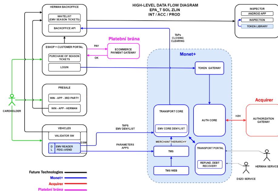
Obrázek 1- blokové schéma systému odbavení
