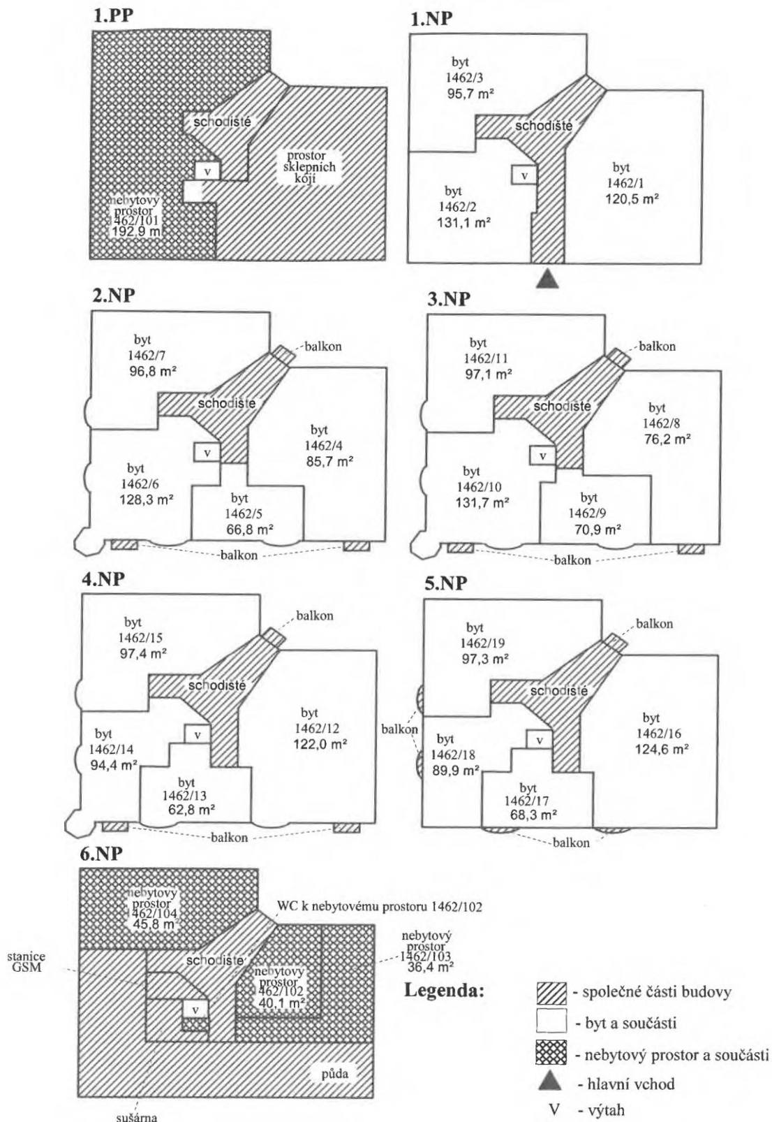
Schema budovy: Kladská č.p. 1462, obec Praha, část obce Vinohrady
