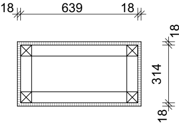
PŮDORYS - ŘEZ SOKLU
