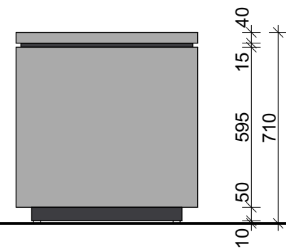
POHLED
