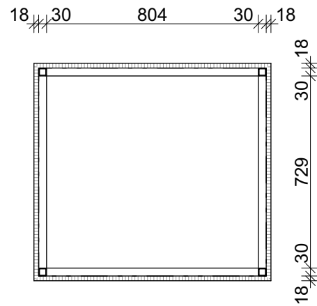
PŮDORYS - ŘEZ SOKLU
