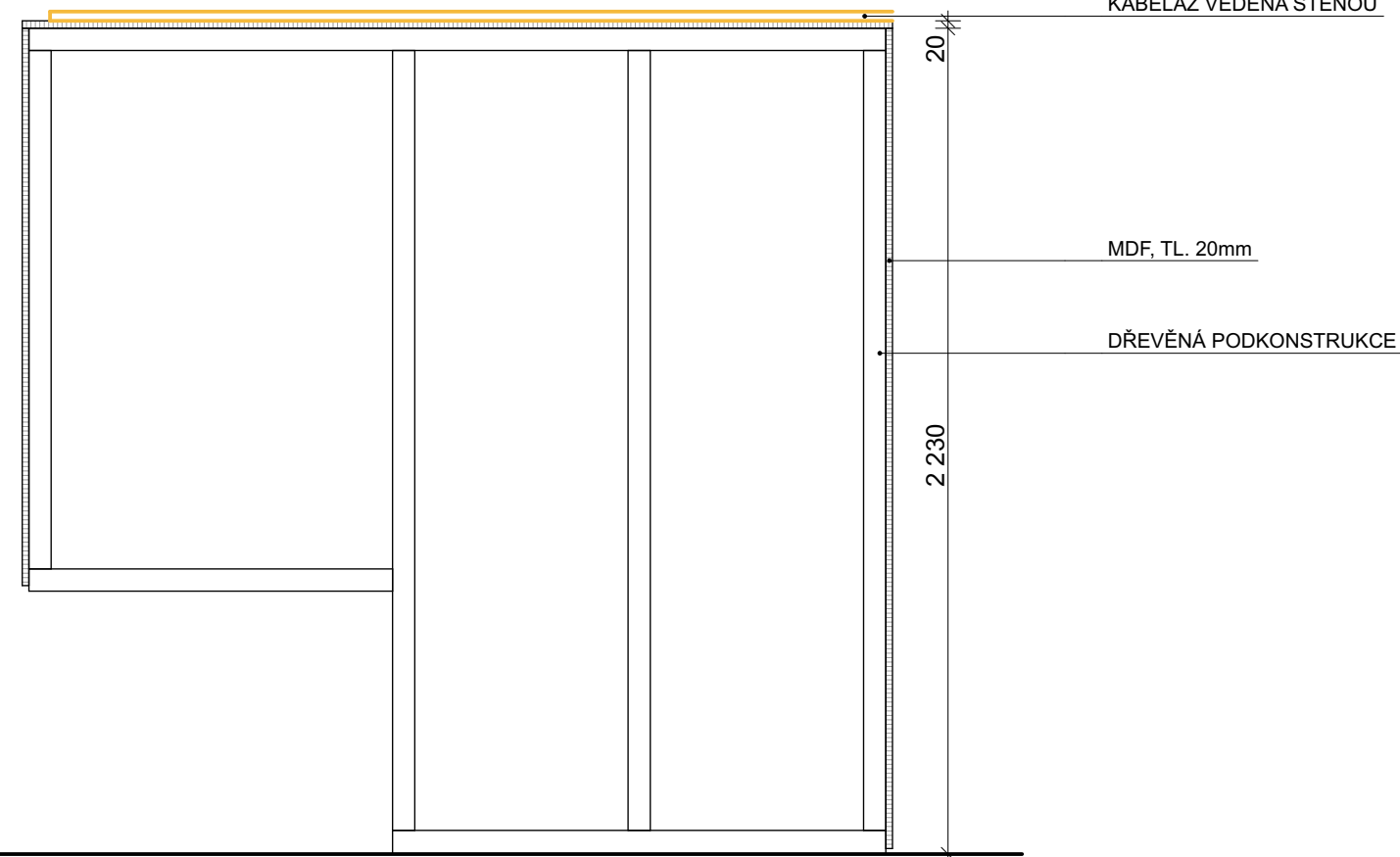
ŘEZ
