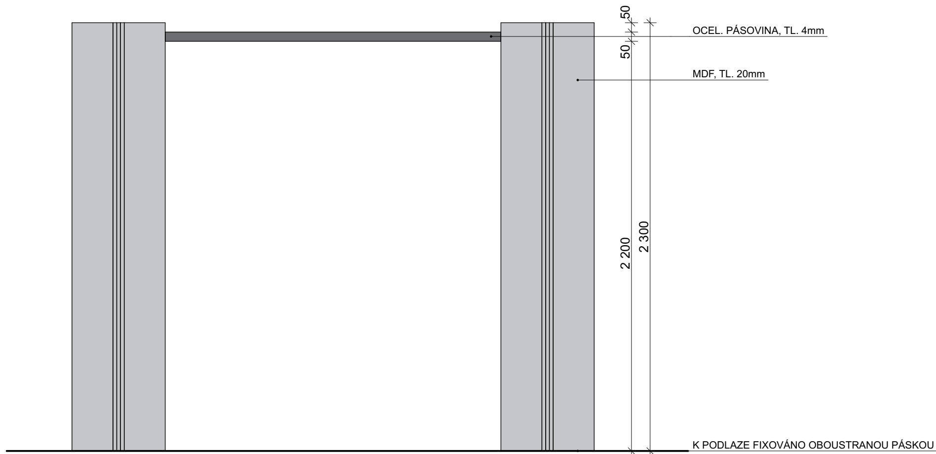
POHLED ČELNÍ
