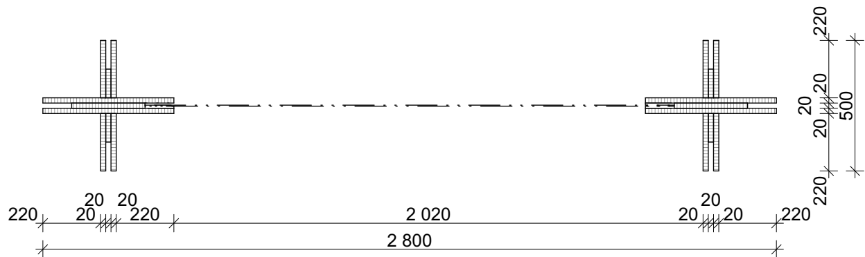
PŮDORYS
