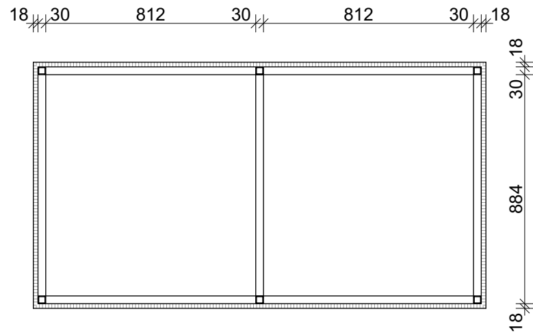
PŮDORYS - ŘEZ SOKLU
