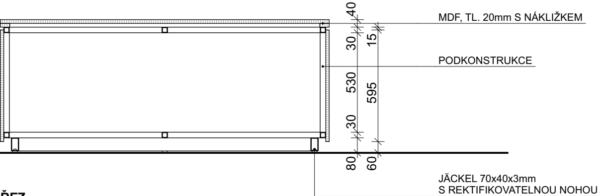
ŘEZ
