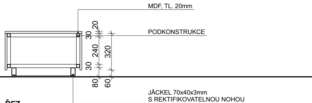
ŘEZ
