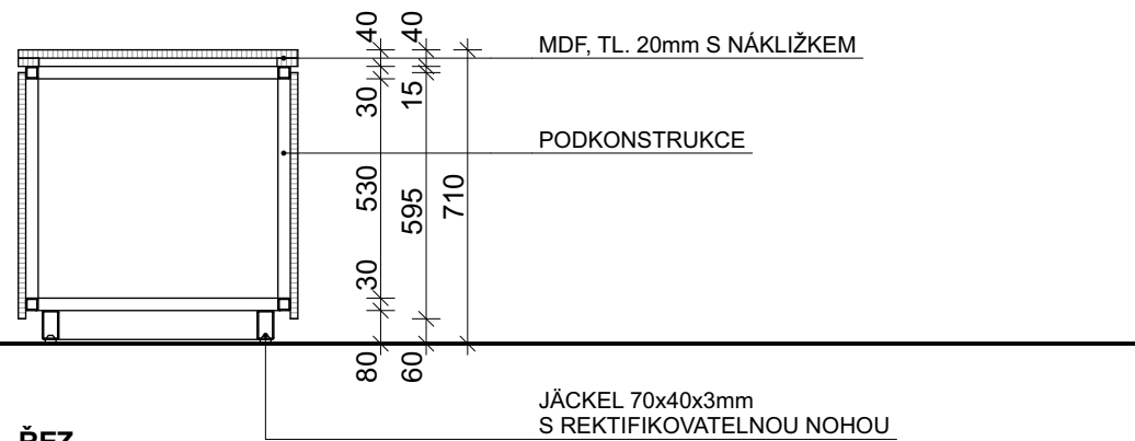
ŘEZ
