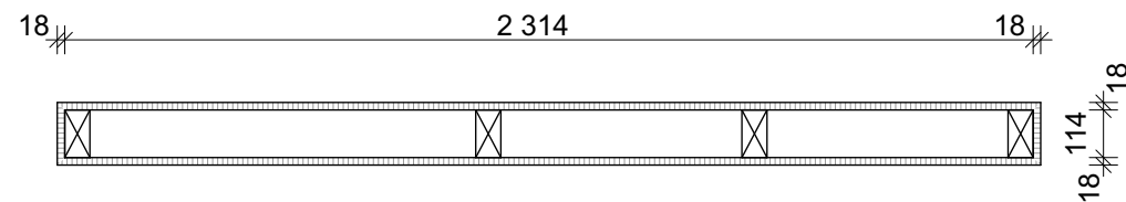
PŮDORYS - ŘEZ SOKLU
