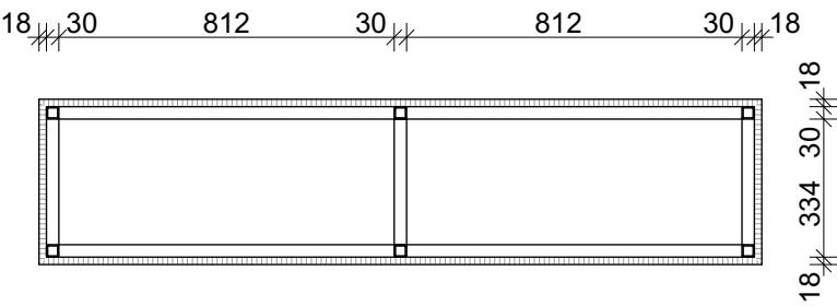
PŮDORYS - ŘEZ SOKLU
