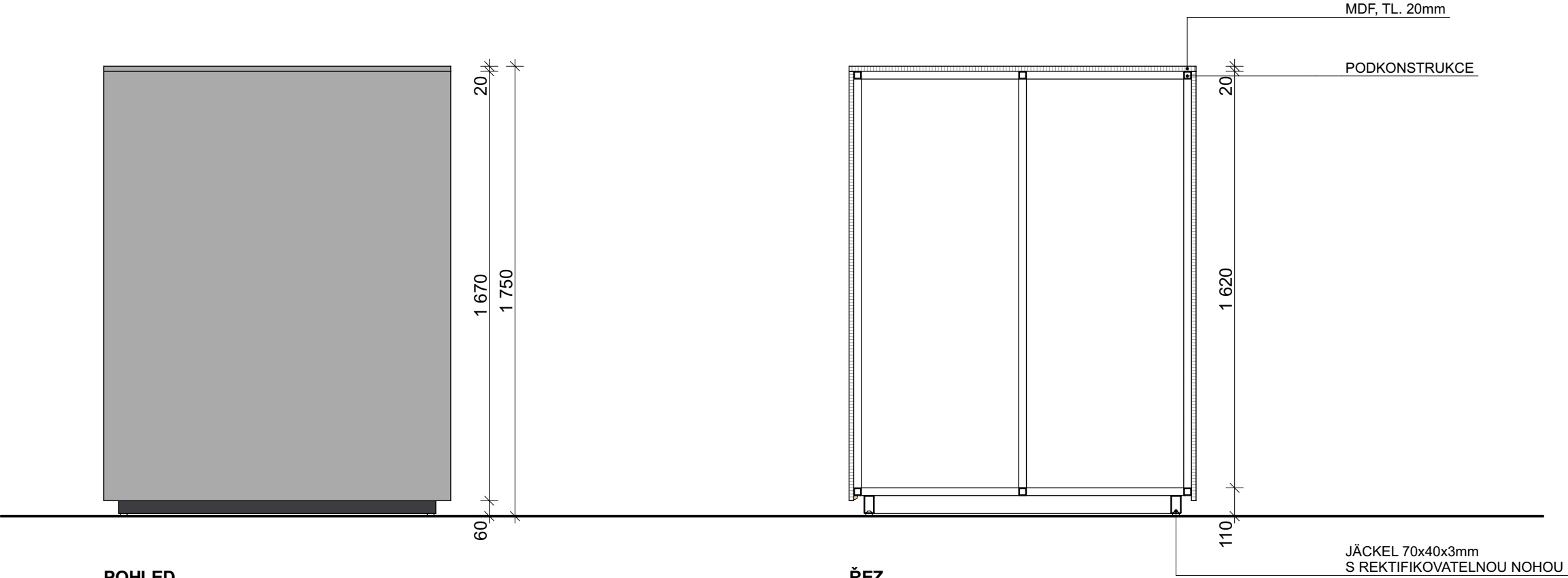
POHLED
