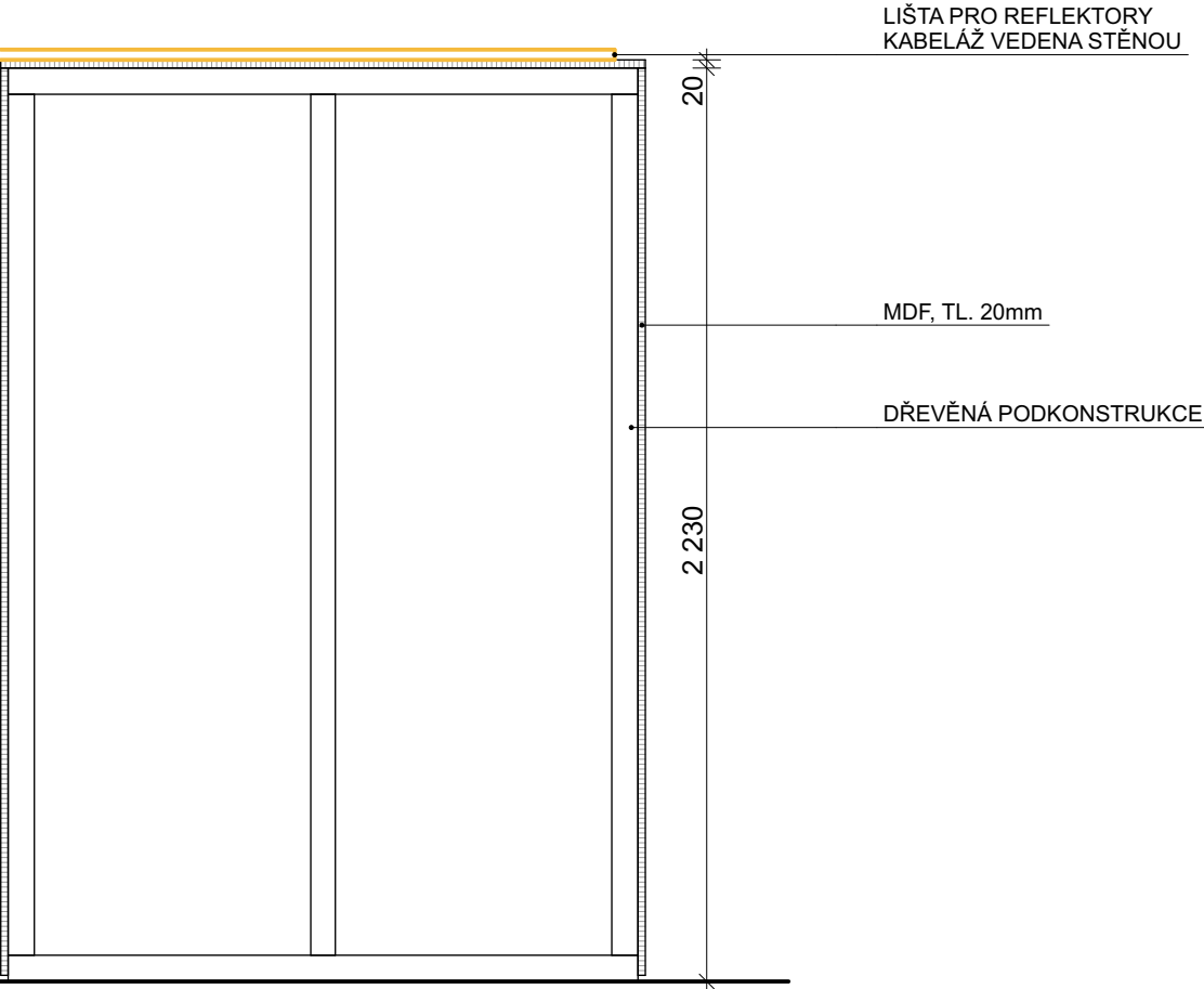
ŘEZ
