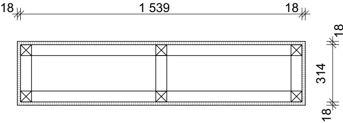
PŮDORYS - ŘEZ SOKLU
