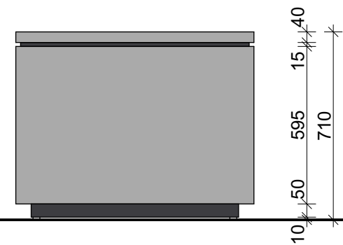
POHLED
