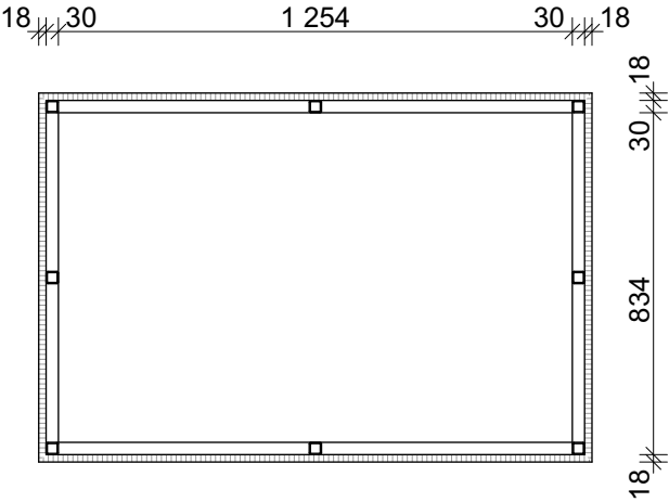
PŮDORYS - ŘEZ SOKLU
