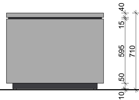
POHLED
