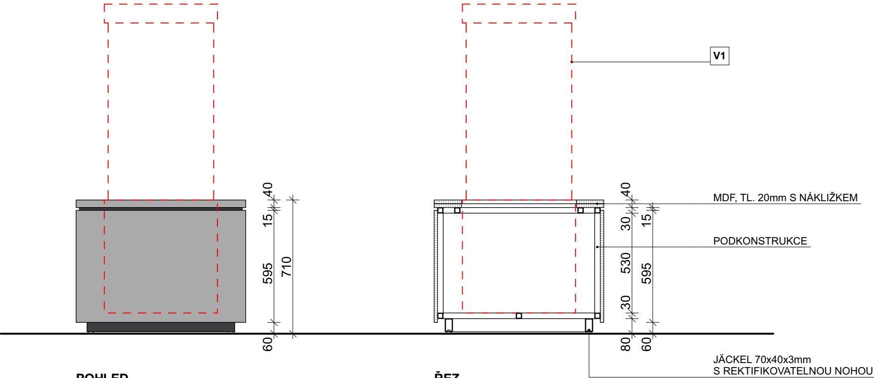
POHLED
