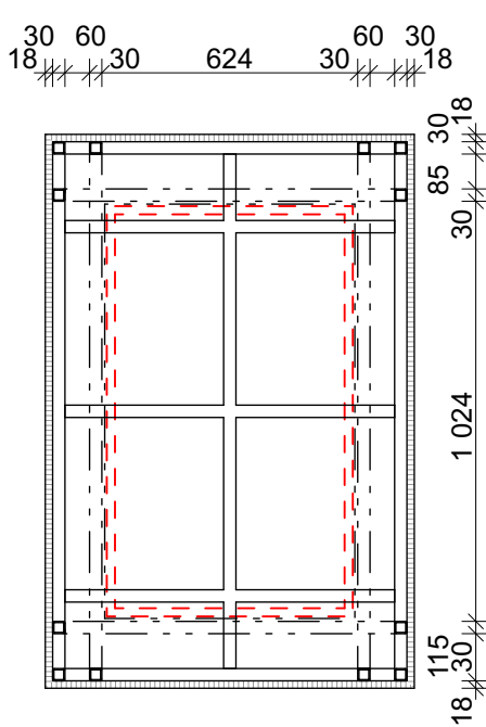
PŮDORYS - ŘEZ SOKLU
