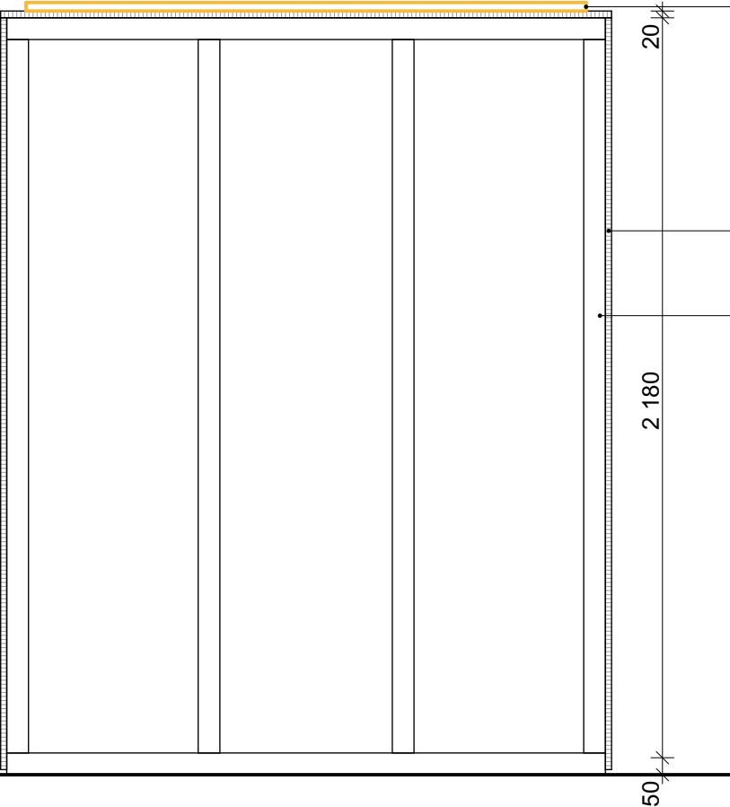
ŘEZ
