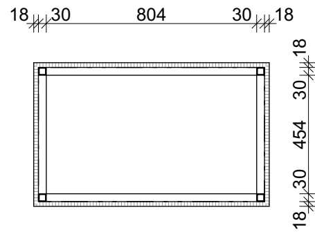
PŮDORYS - ŘEZ SOKLU
