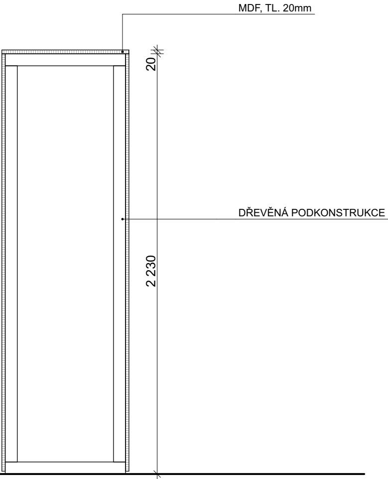
ŘEZ
