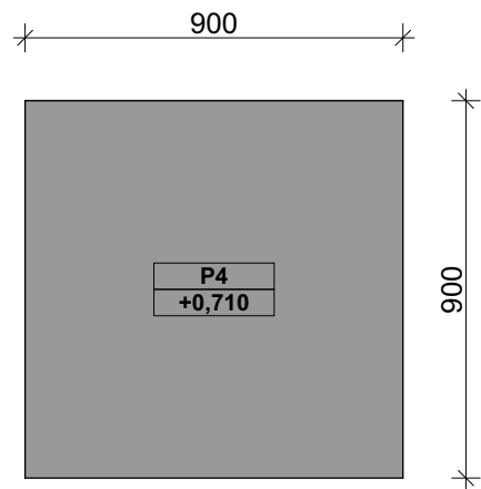
PŮDORYS
