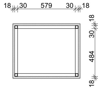
PŮDORYS - ŘEZ SOKLU
