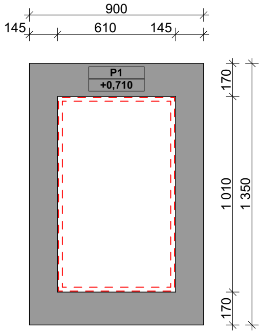
PŮDORYS
