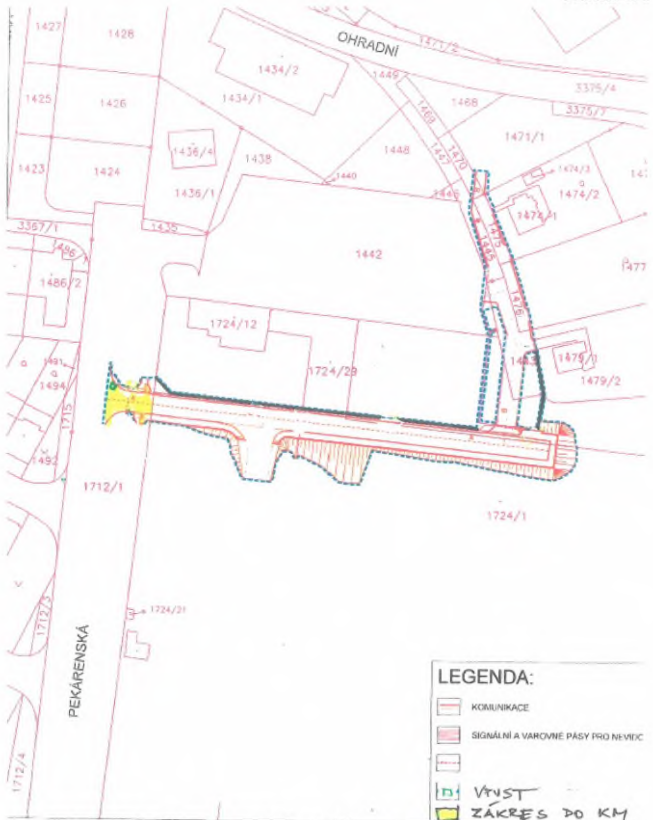
SITUACE - VYJEZD Z PŘELOŽKY KOMUNIK. PEKÁRENSKÁ
