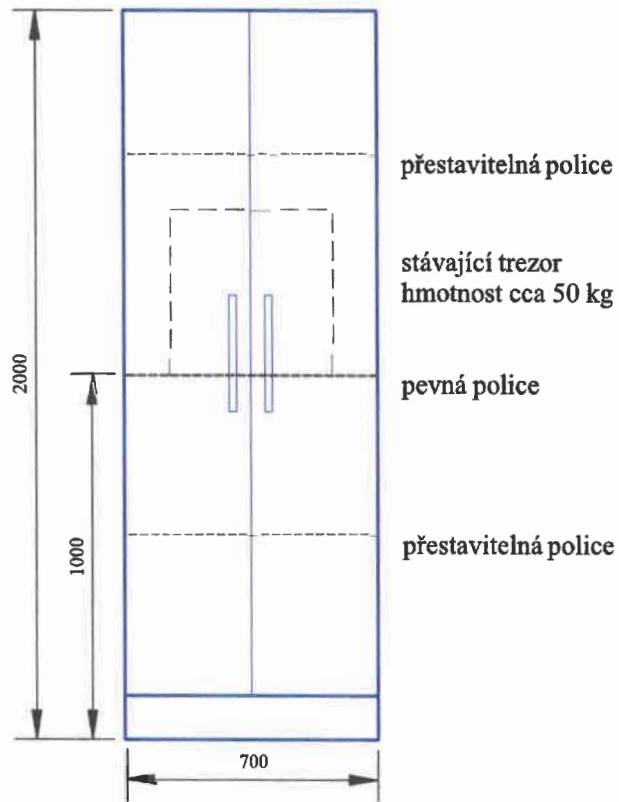
skříň na trezor
