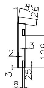
ŘEZ A-A
