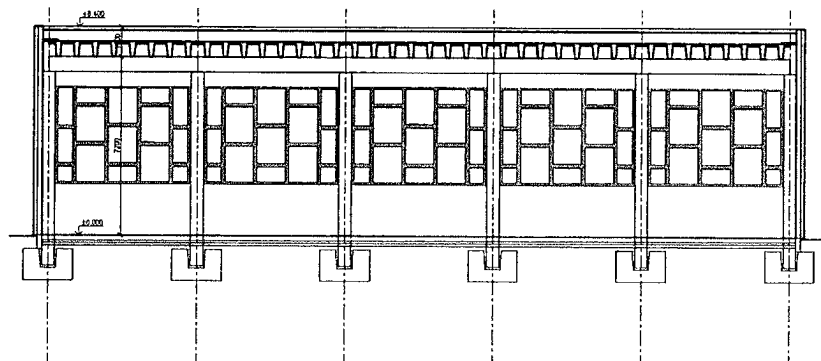
Řez A - A` (1 : 200)
