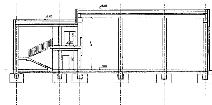
Řez B - B` (1 : 200)
