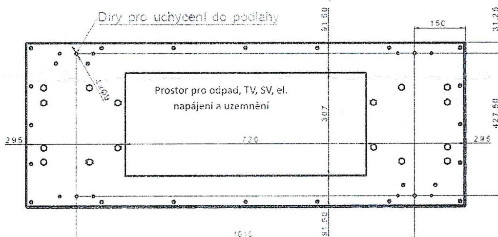
Detail základové desky
