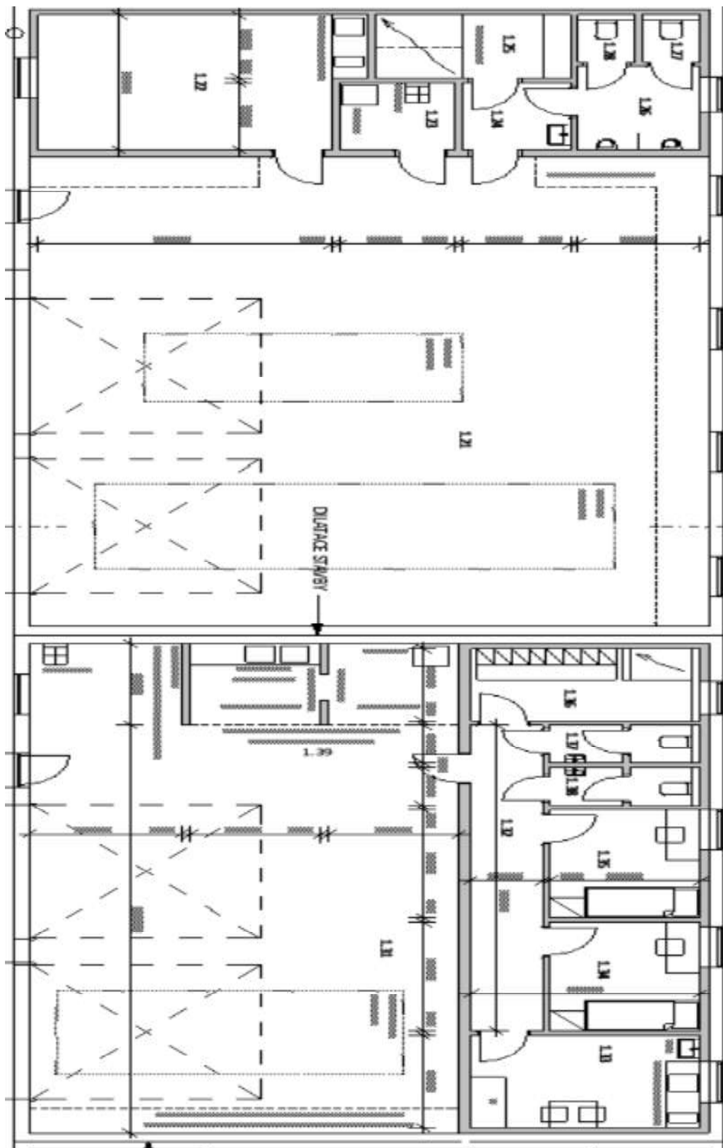
Příloha č. 3 - situační plánec stavby včetně vestavby zázemí
