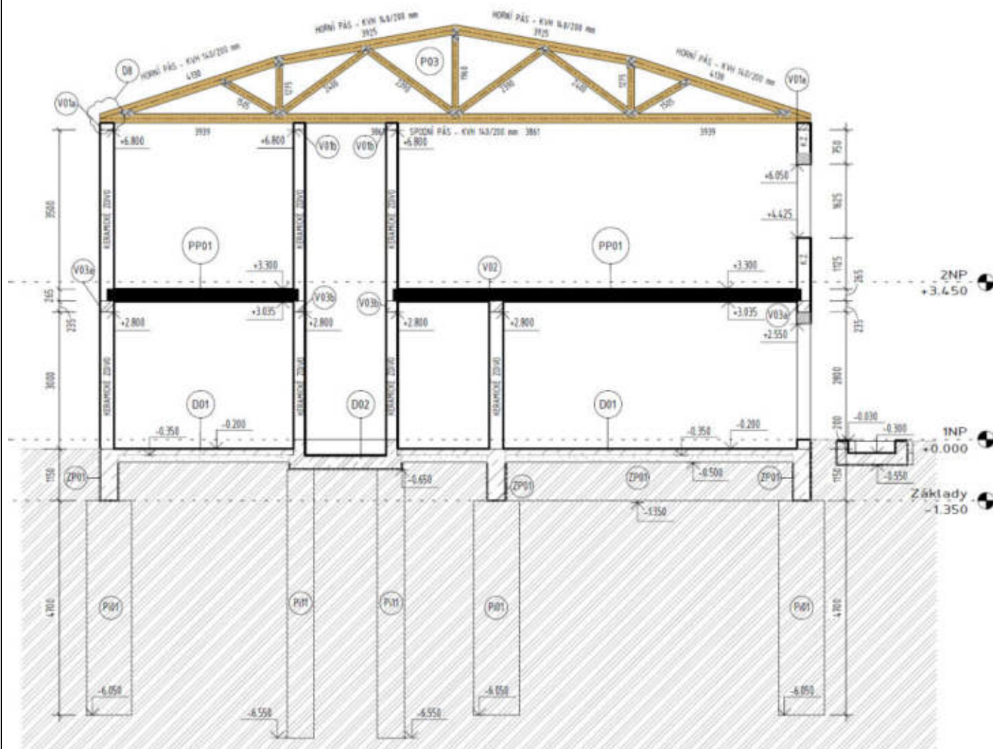
Typický příčný řez objektem, obvodové stěny v tloušťce 300 mm bez jakéhokoli ztužení
