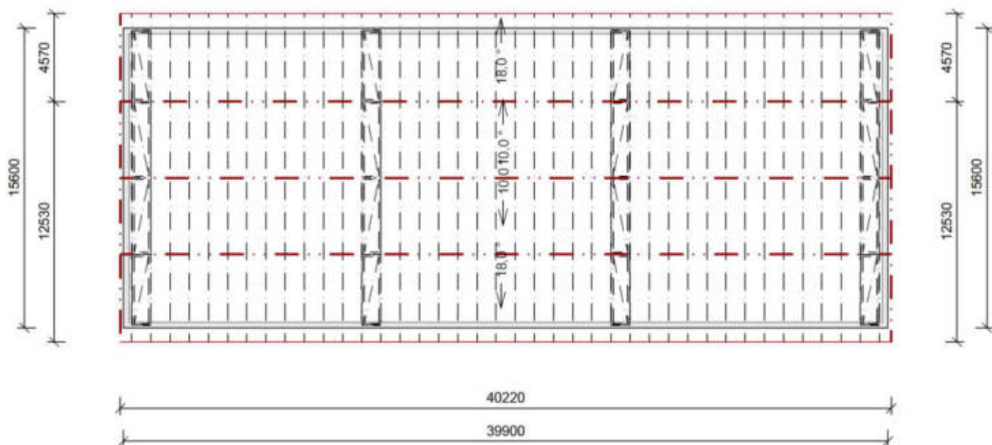
Půdorys nosné konstrukce střechy
