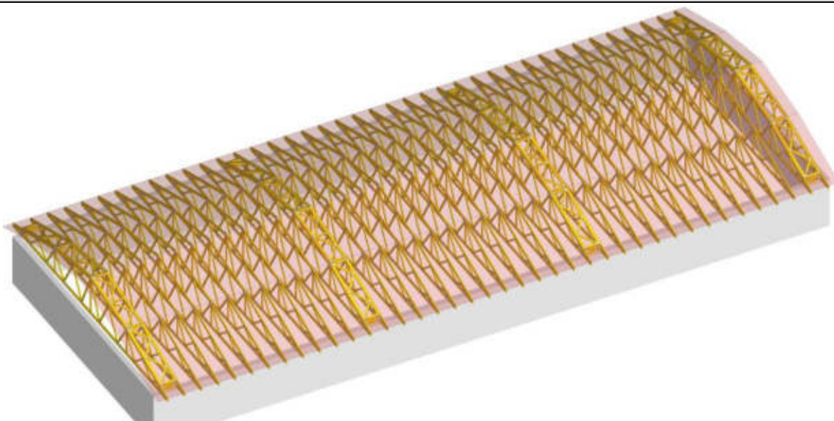
Axonometrie nosné konstrukce střechy
