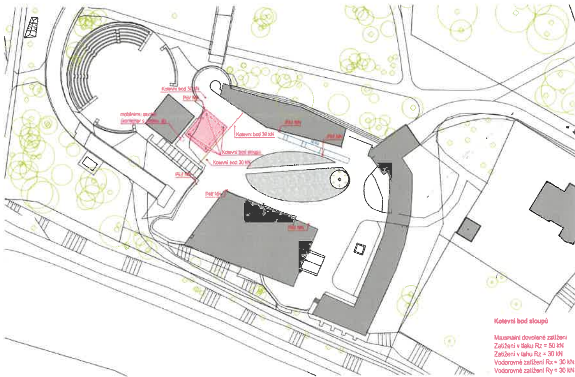
Pozice 1 dočasného podia 10x8 m, M 1:750
