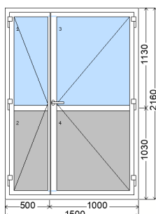
dveře vnitřní pohled (interiér)
