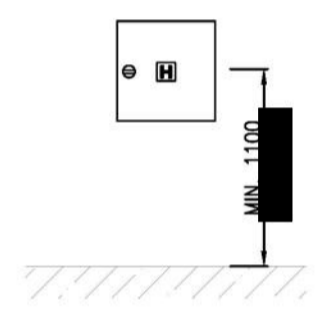
UMÍSTĚNÍ HADICOVÉHO SYSTÉMU (1:50)
