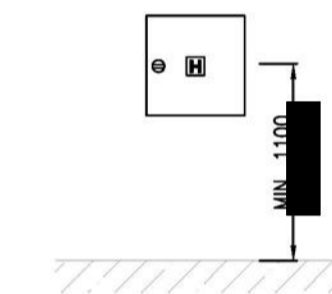
UMÍSTĚNÍ HADICOVÉHO SYSTÉMU (1:50)
