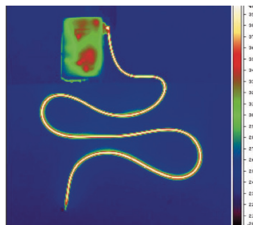
rovnoměrný ohřev po celé délce setu HOTLINE®
