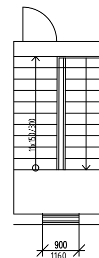
3.NP
