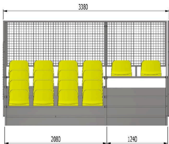
Rozměry čtyřradé tribuny
