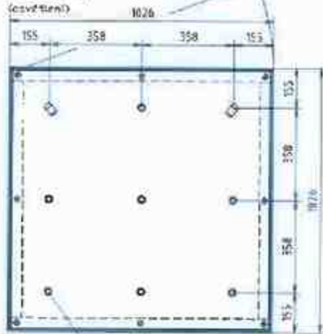
Řez B-B: (souvřítí)
