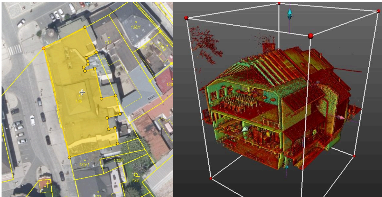
Obrázek 1 3D mračno bodů budovy
