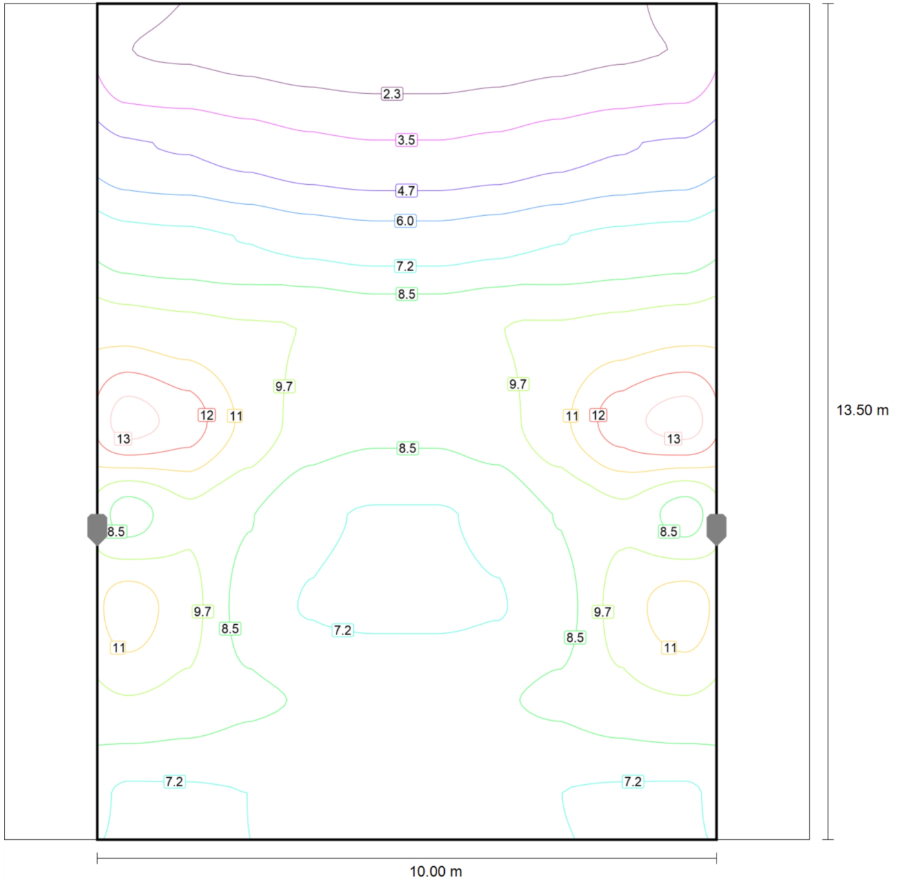
Hodnota údržby "Horizontální intenzita osvětlení" [lx] (Čáry Isolux)
