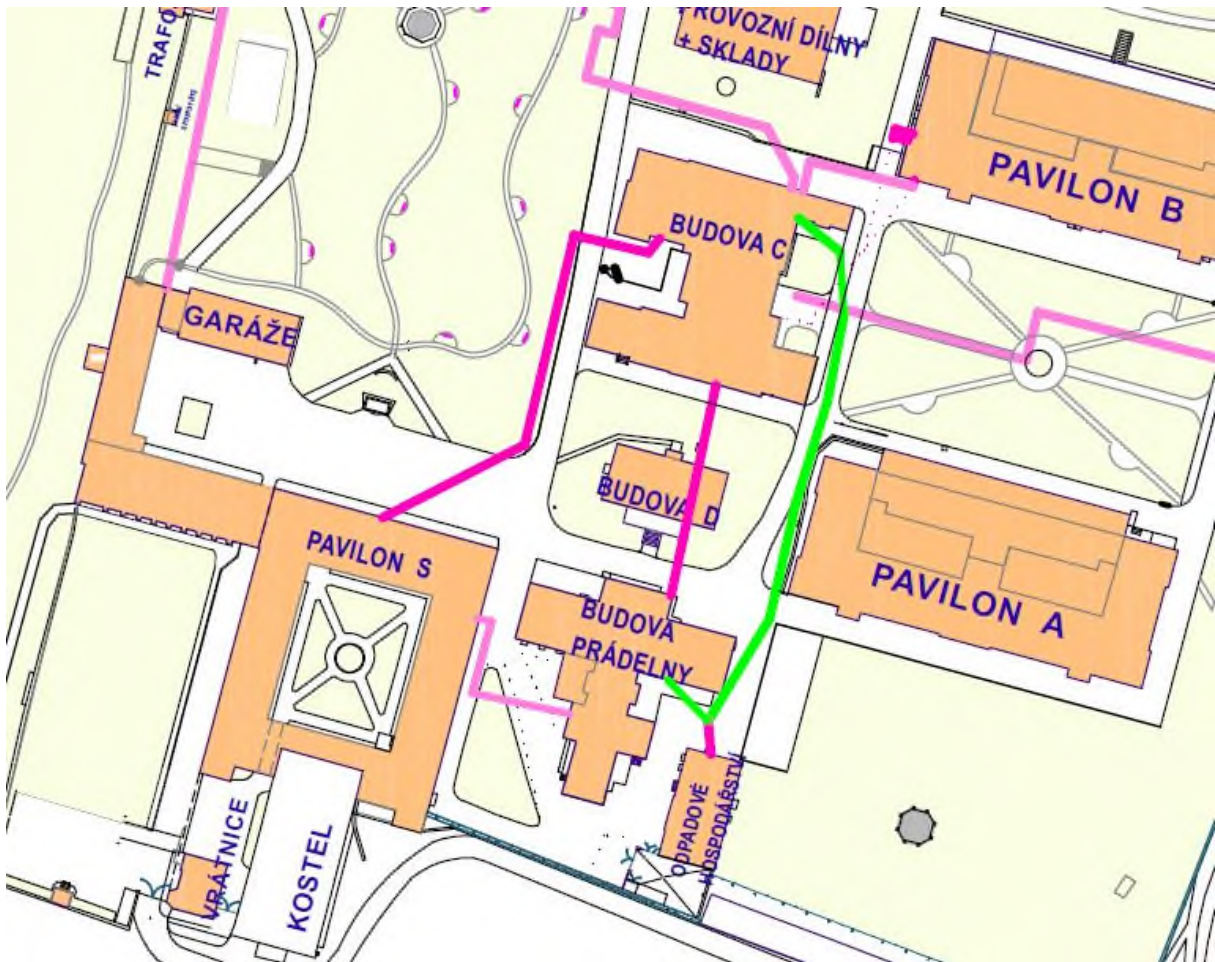
Obrázek 2: Rozvod podzemního parovodu z kotelny K1 do budovy prádelny
