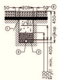
A2) Chodník (povrch - dlažba/asfalt)
