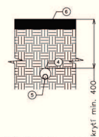
C3) Podvrt vozovka (dálnice, silnice pro motorová, vozidla, silnice I. tř., II. tř., III. tř.) Podvrt drážní tělesa (tramvaj, trolejbus)
