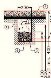
A3) Chodník (povrch - beton)
