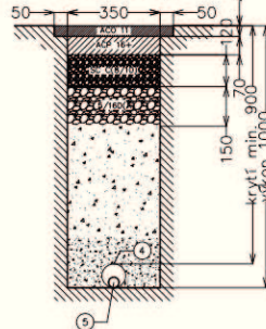
C) Přečody vjezdů a komunikací C1) Vozovka (místní a účelové komunikace)
