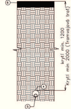
C3) Podvrt vozovka (dálnice, silnice pro motorová, vozidla, silnice I. tř., II. tř., III. tř.) Podvrt drážní tělesa (tramvaj, trolejbus)
