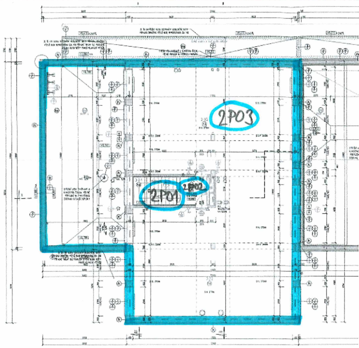
PŮDORPE 1.NP - VYPRÁVNÍ BUDOVA
