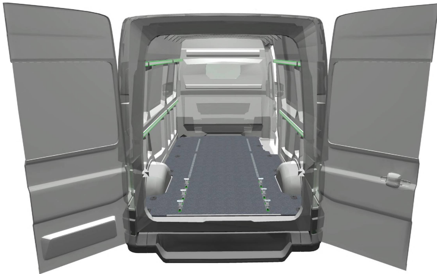
Volkswagen Crafter (2016) L4 H3 Vyska nakladači hrany: cca 570 mm
