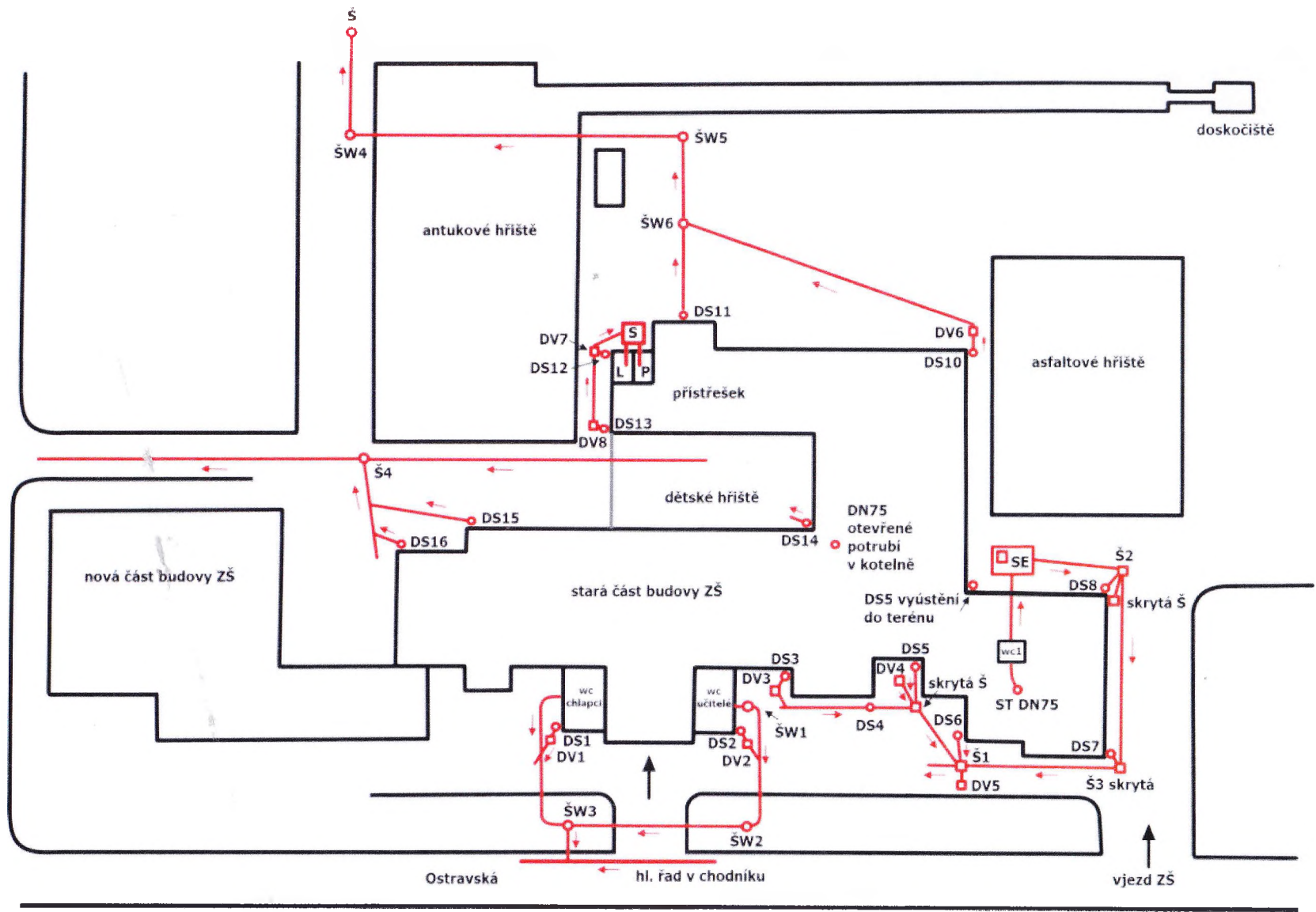
Schéma splaškové a dešťové kanalizace ZŠ a MŠ T. G. Masaryka, Ostravská 658/28, Bílovec
