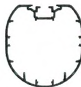
Profil rámu branky 105 x 100 mm
