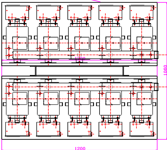
Obrys kotle
