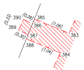
Detail:AG
