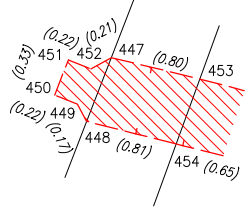
Detail:AK
