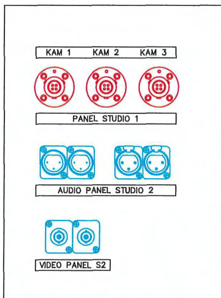
Připojný panel venkovní pocha
