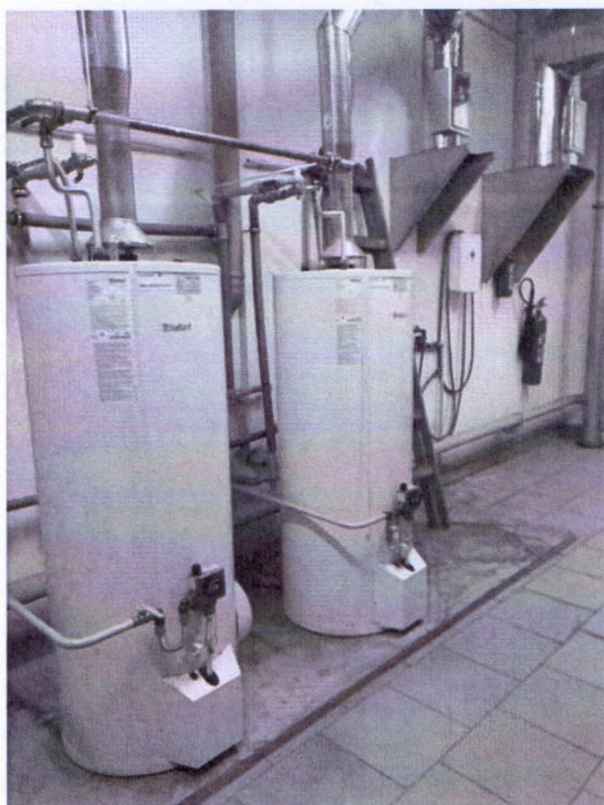
Plynové boilery na ohřev TUV v kotelně ve 5.NP
