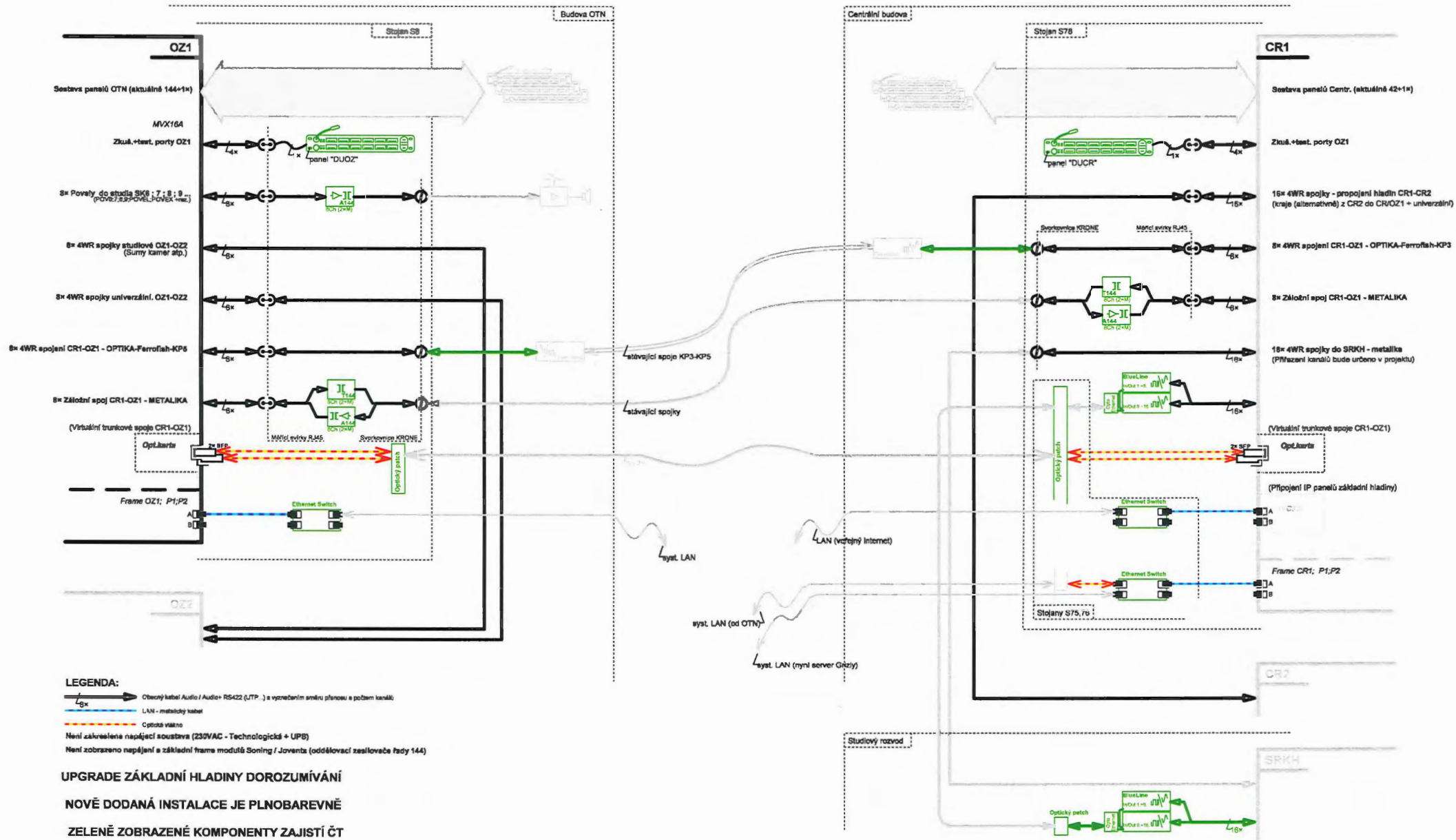
PŘÍLOHA 2b - SCHEMA PROPOJENÍ SIGNÁLŮ
