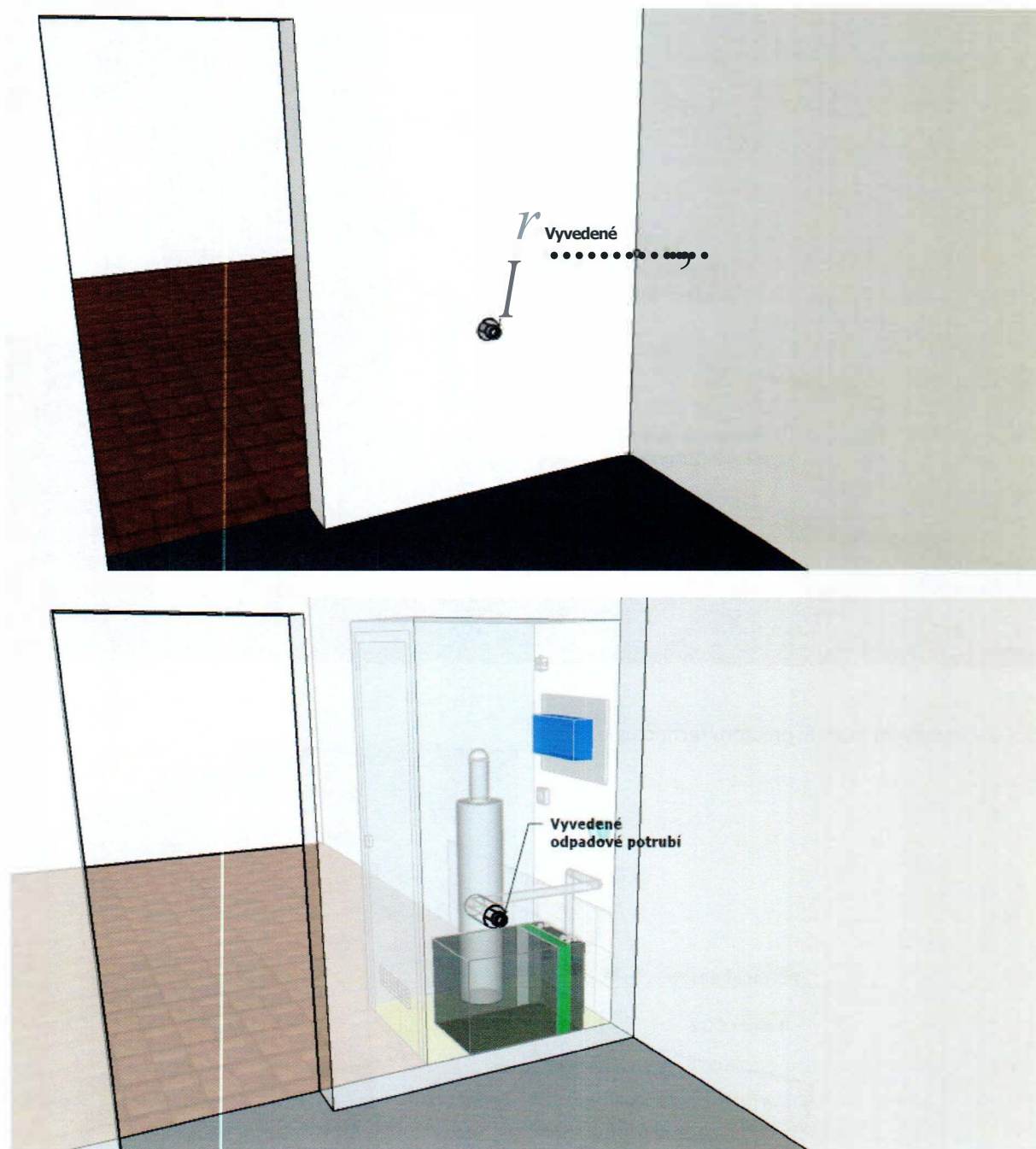
Obr. 6,7 -vyvedené odpadové potrubí
