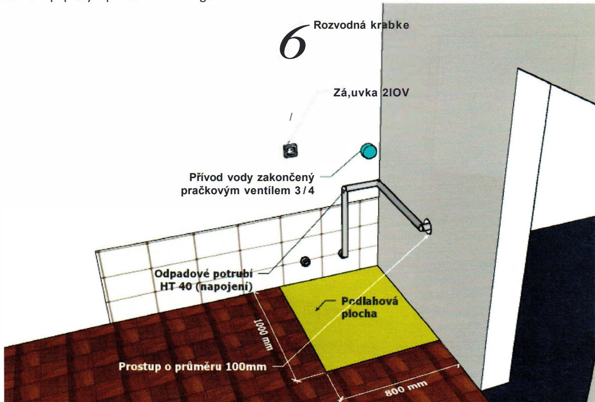
Obr. 4 - přípravy v prostoru technologie
