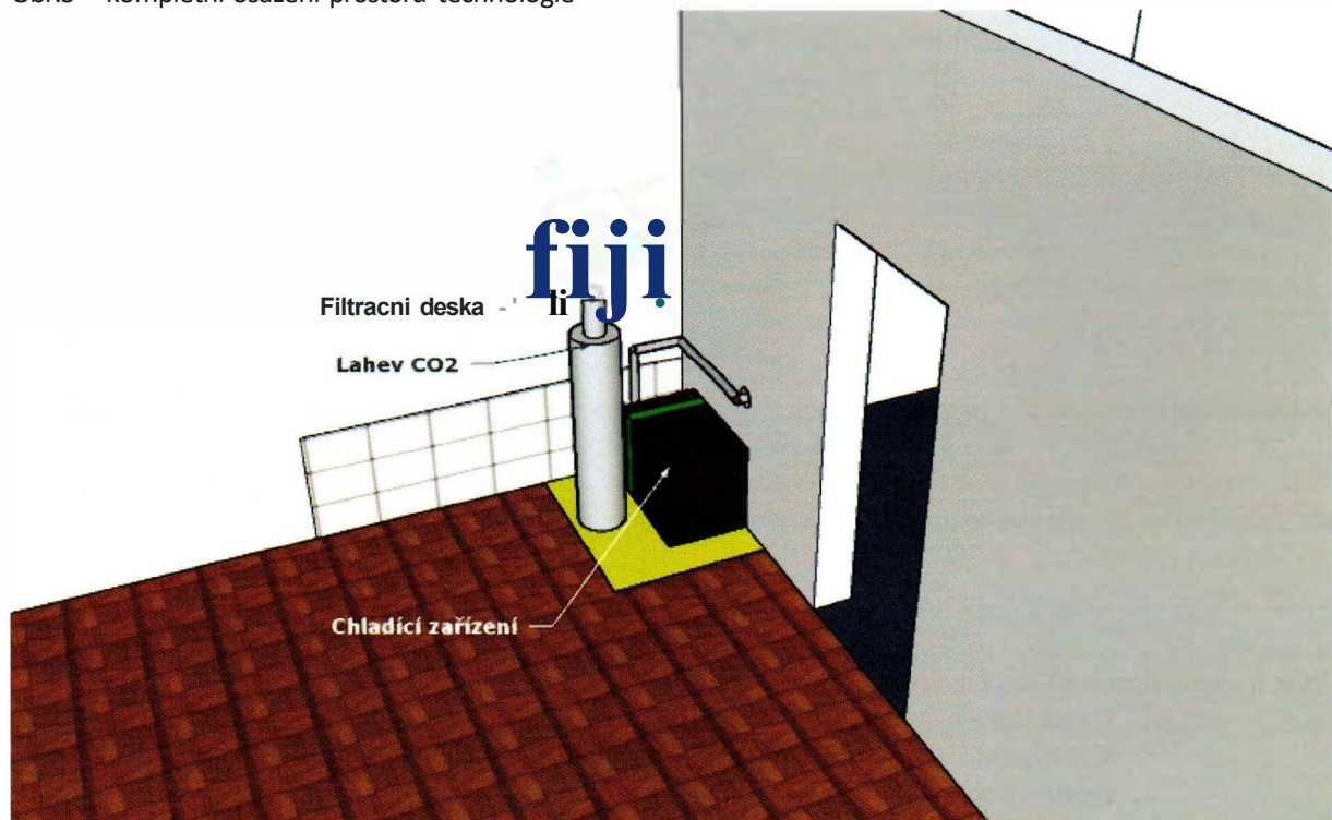
Obr.S - kompletní osazení prostoru technologie
