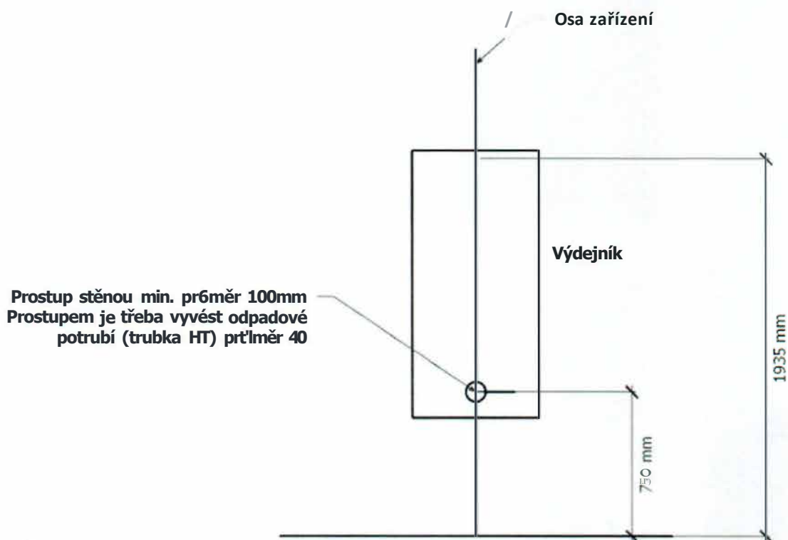
Obr. 3 - Šablona prostupu přímo na stěně
