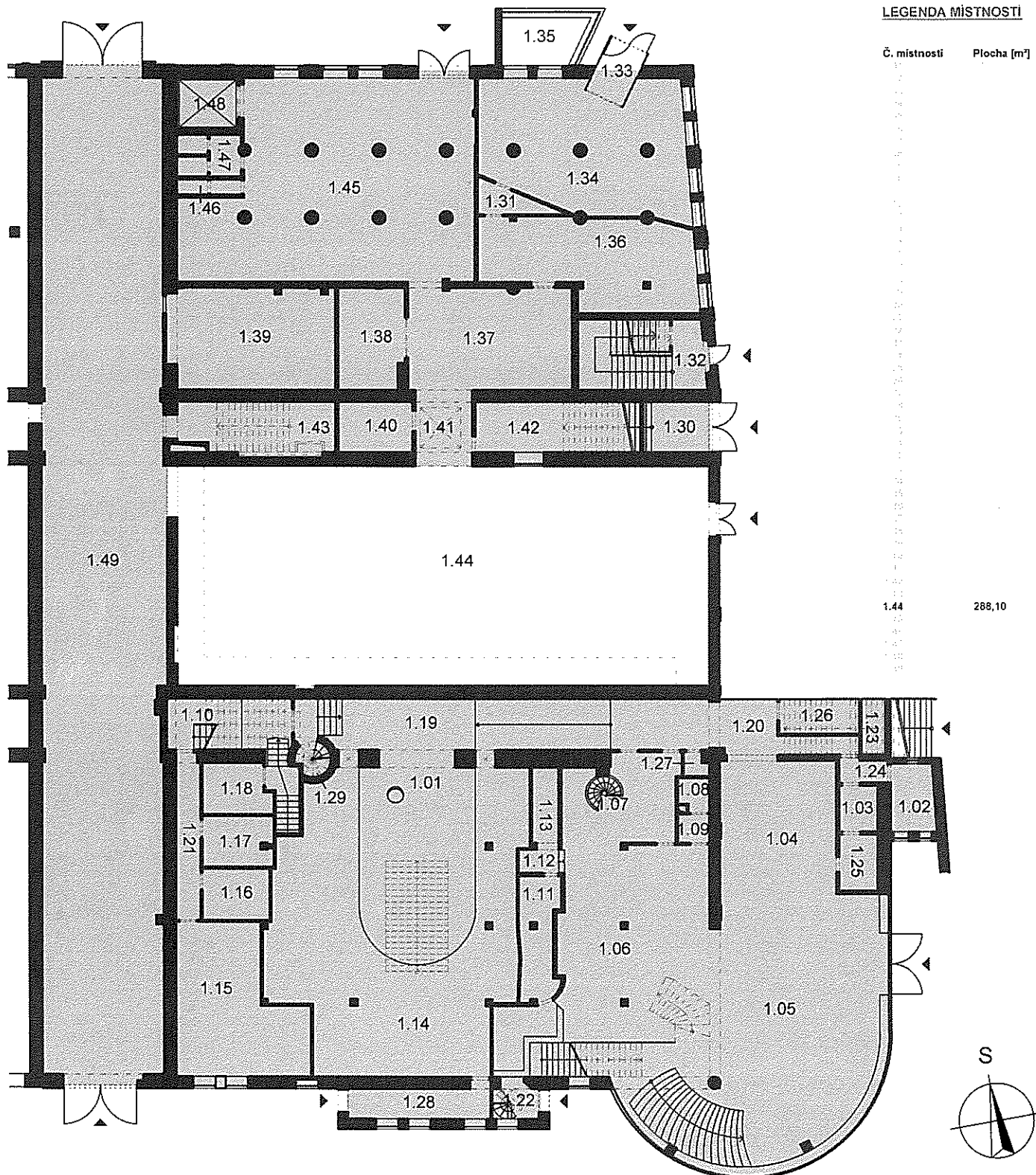
Schematický půdorys 1.NP
