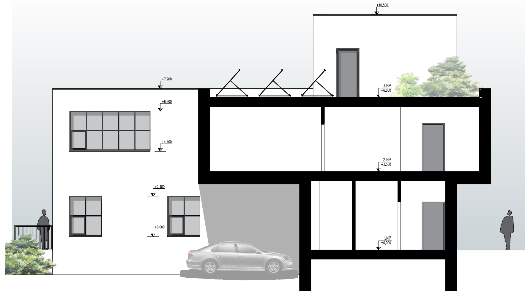
ŘEZ A-A'
