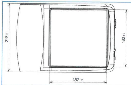
Technický výkres s rozměry vah Entris II Essential s dílkem 0.1 g
