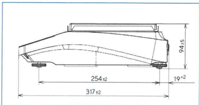
Technický výkres s rozměry vah Entris II Essential s dílkem 0.1 g
