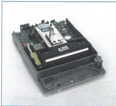
foto monolitického bloku s uložením vážního systému pro váhy Entris II ukotvení systému v duralové základně činí váhu rychlou a stabilní
