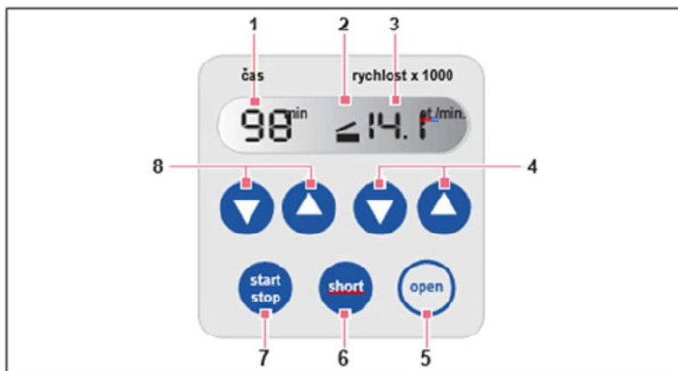
obr. 5-1: Ovládací prvky obsluhy – MiniSpin / MiniSpin plus
