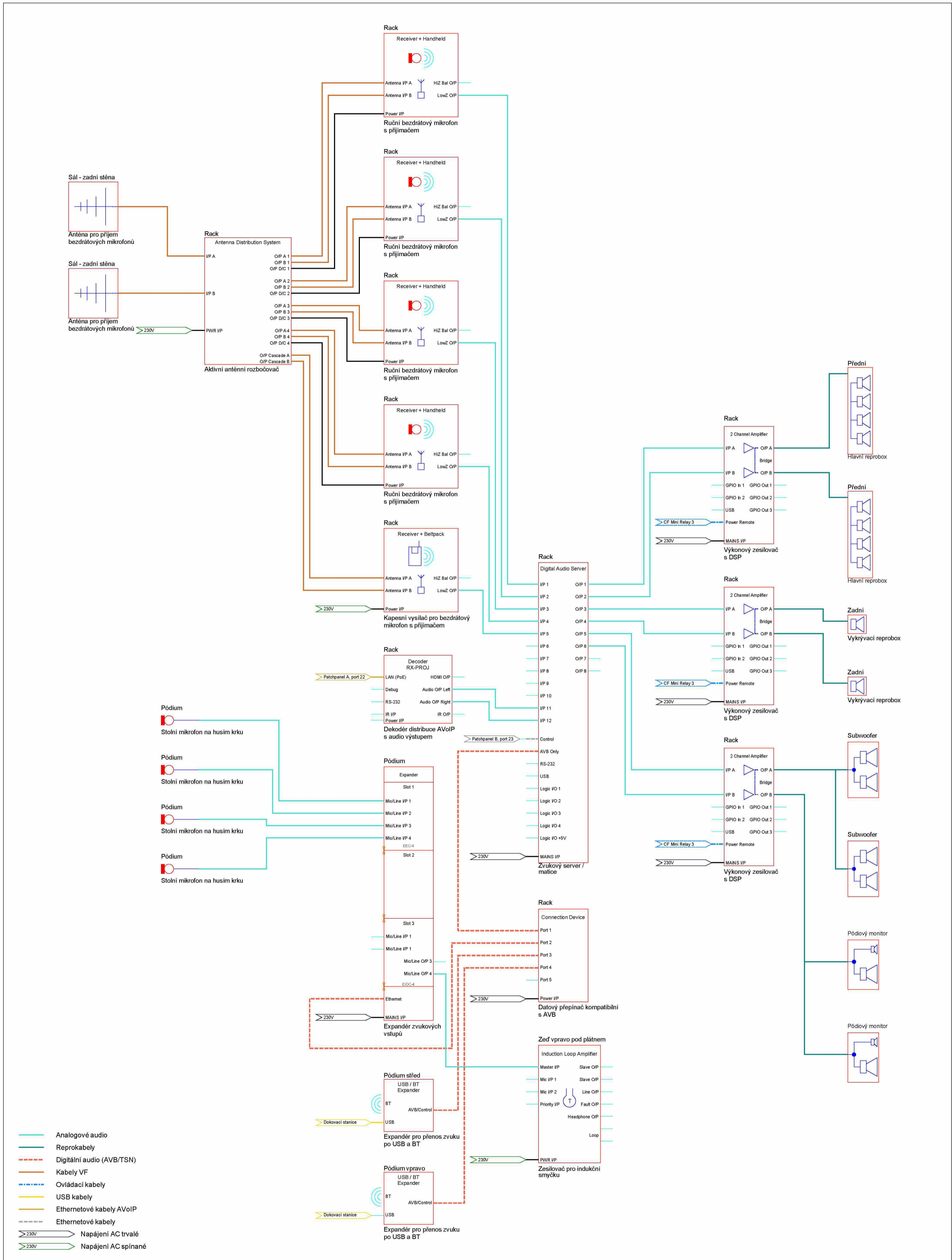
Název Multifunkční sál - schéma Audio
