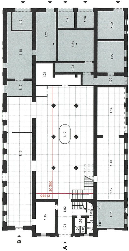
SCHEMATICKÝ PŮDORYS 1.NP
