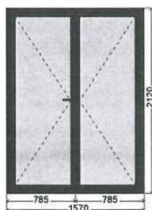
dveře ven otvíravé vnější pohled (exteriér)
