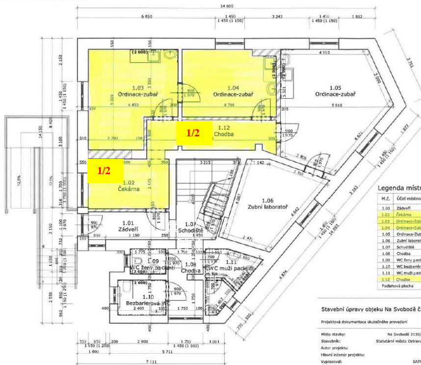
Půdorys 1.NP skutečné provedení
