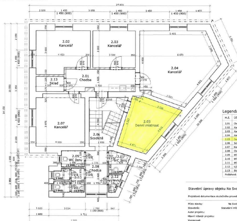
Půdorys 2.NP skutečné provedení
