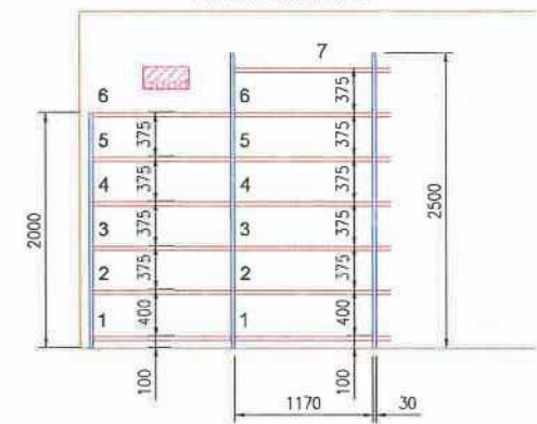
VÝŠKOVÉ ČLENĚNÍ S1
