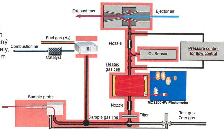
Obr. 2 Schéma analyzátoru MCS200HW
