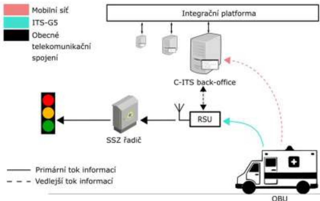
Obrázek 31: Schéma fungování služby EVA – prioritita SSZ
