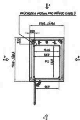
PŮDORYS V ±0
