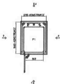
PŮDORYS V +3820
