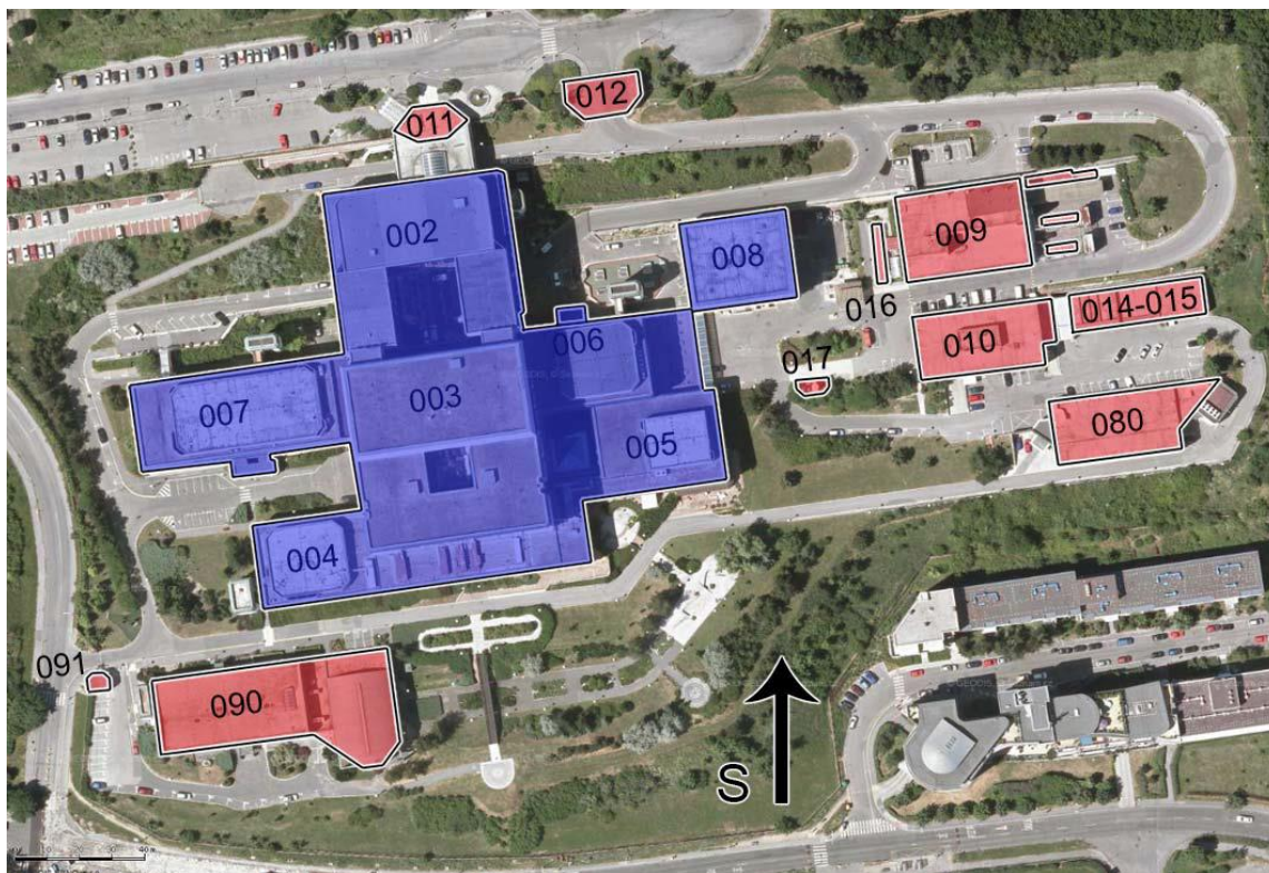
Obr. č. 3-1 – Situace Areálu NEMOCNICE NA HOMOLCE
