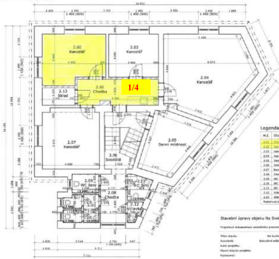
Příloha 2.NP skutečné provedení
